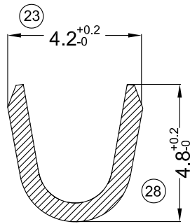
SECC. A-A
