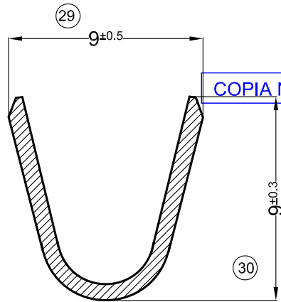
SECC. B-B
