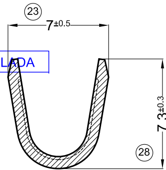
SECC. A-A
